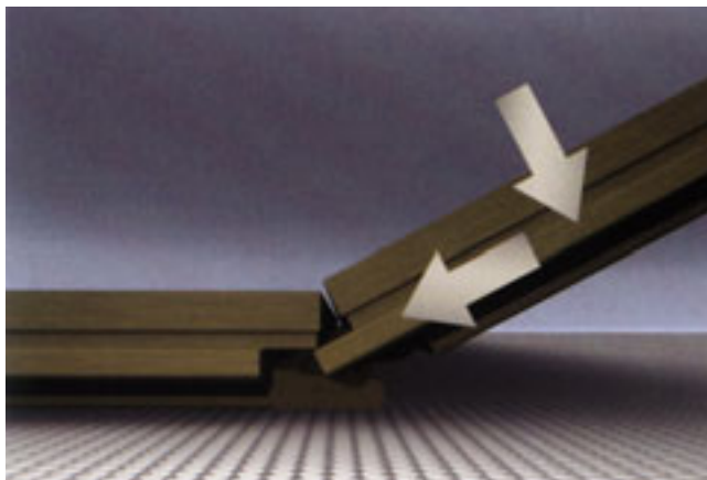
Método 1: Girar y ensamblar con un clic
